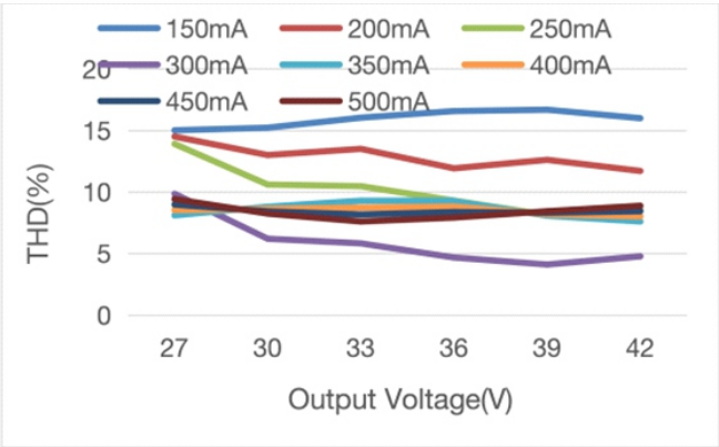
Зависимость полного гармонического искажения от выходного напряжения
